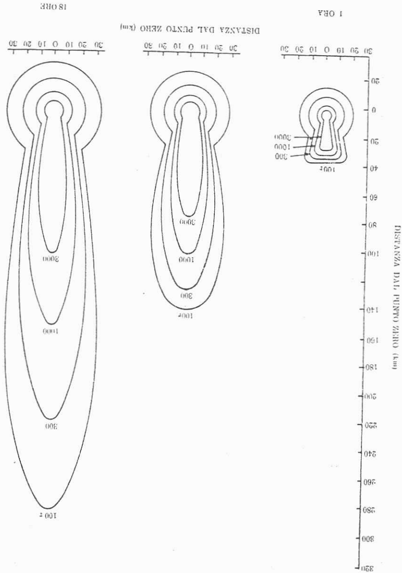
Fig. 7 - Linee isodose ad 1, a 6 ed a 18 ore dopo l'esplosione in superficie di una bomba a fissione di energia dell'ordine del Mt (velocità del vento efficace 23 chilometri all'ora).
